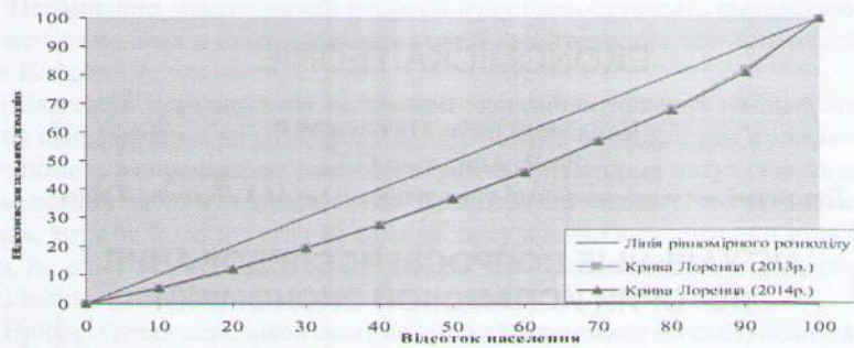
Рис.4. Крива Лоренца
