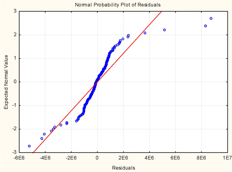
Рис. 5. Нормальний імовірнісний графік залишків моделі для експорту
