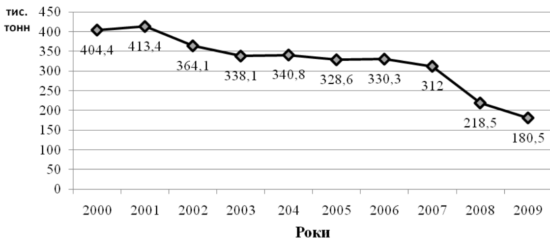
Рис. 2. Задіяна потужність цукрових заводів України
