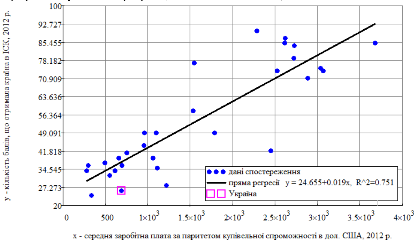
Рис. 2. Діаграма розподілу і пряма регресія для показників CPI та «середня зарплата за ПКС»*
