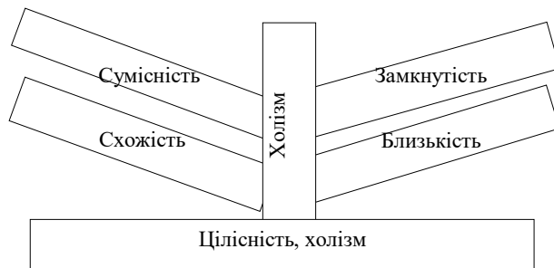
Рис. 3. Дерево гешталту
