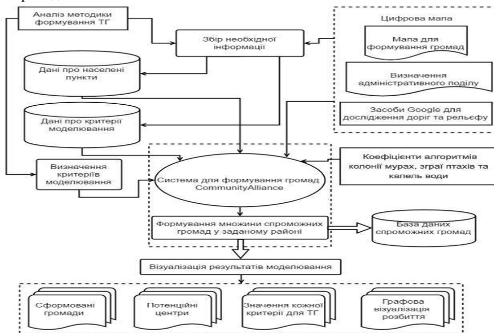
Рисунок 1 – Логічна структура програмної реалізації системи формування громад
