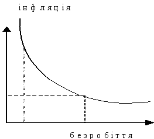
Крива Філіпса [3]
