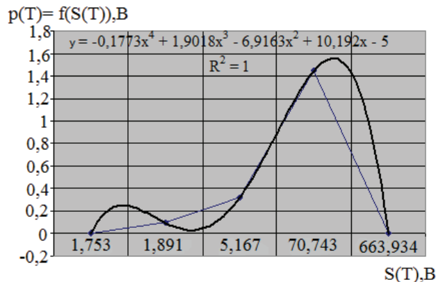
Рис. 6. Температурна залежність поправок вихідного сигналу для забезпечення лінійності функції перетворення ОПС ТМВ у діапазоні температур 692,677 \div 1357,77 К та спектральній смузі 1 \div 2 мкм
