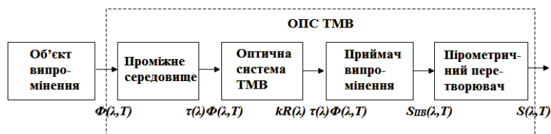
Рис. 2. Загальна схема впливу складових ОПС ТМВ на перетворення сигналу випромінення об'єкта в нормований електричний сигнал
