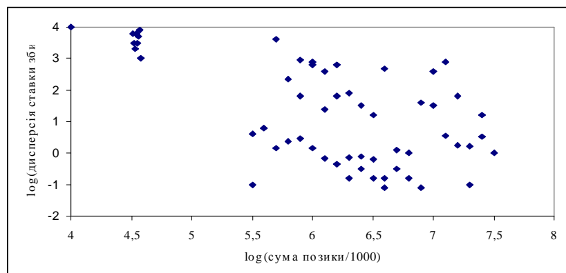
Рис.1. Залежність дисперсії ставки збитків кредитного портфеля від обсягу споживчого кредитування в ньому
