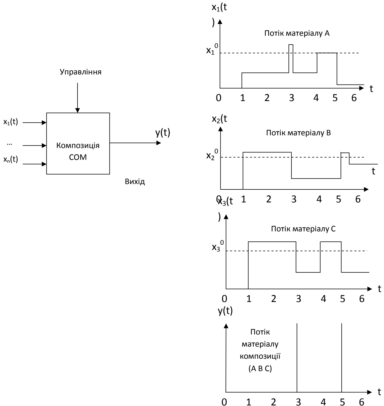
Рис.3.7. Перетворення «композиція потоків»
